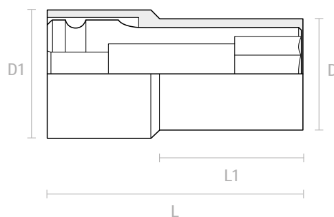
Nástrčná hlavice dvojité 6-ti hran L60/65, Pinch-point 12-point socket L60/65, Pinch-point
