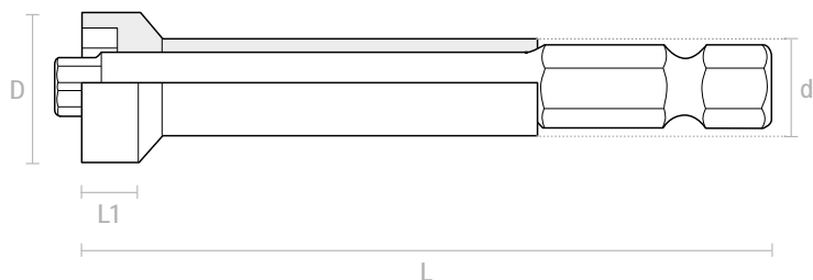
covertec Bit s přídržnou funkcí, pevné pouzdro, Torx covertec Bit with holding function fix shell, Torx
