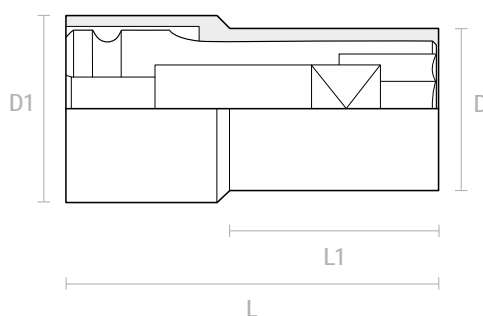
Nástrčná hlavice 6-ti hranná s tyčovým magnetem 1", Pinch-point 6-point socket with central magnet 1", Pinch-point
