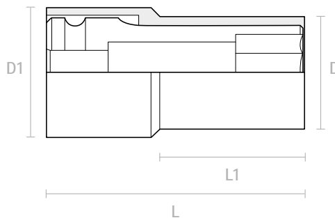
Nástrčná hlavice Surface-drive L80 Socket surface-drive L80
